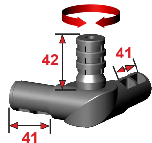
3D3R30X2(3)K/GELENK
