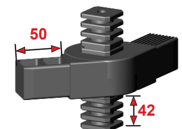
3D4V40K/GELENK/180°
