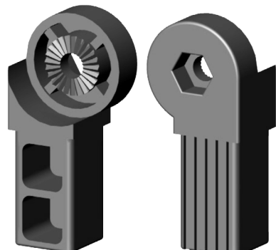
Arretiermöglichkeit in 15°-Schritten stop in steps of 15° dispositif d'arrêt en pas de 15°
